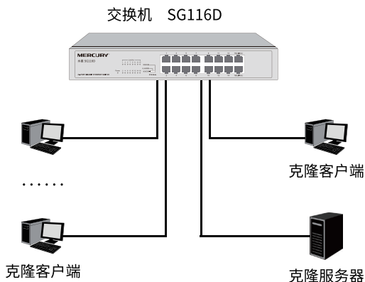
图2-3 网络克隆模式拓扑示例
